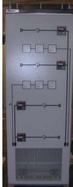
Niederspannungsschaltanlage Typ GNS-KVS
